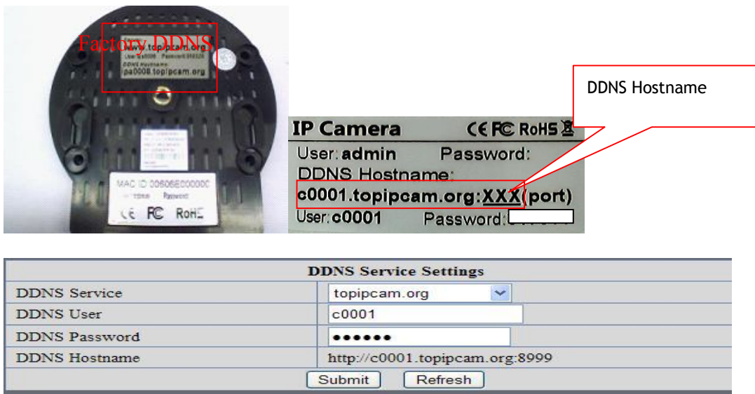
Figura 73 DDNS de fábrica.
